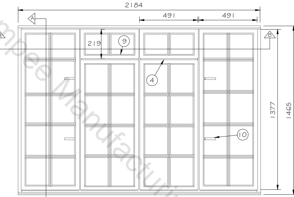
FRONT ELEVATION SCALE: 1:20
