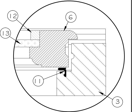
DETAIL-B SCALE: 1:2
